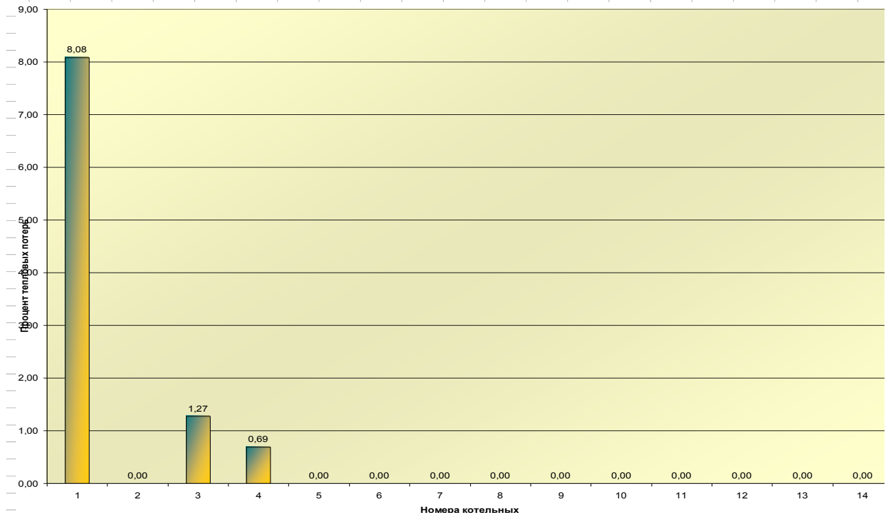
Потери ( % ) тепла через теплоизоляционную конструкцию трубопроводов теплосети ( по котельным № 1 -- 6 )
