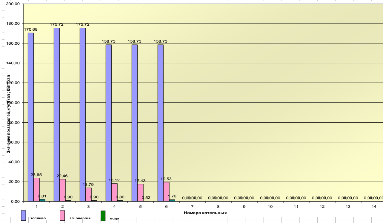
Значения удельных расходов топлива, эл. энергии и воды на выработку 1 Гкал тепловой энергии ( по котельным № 1 -- 6 )
